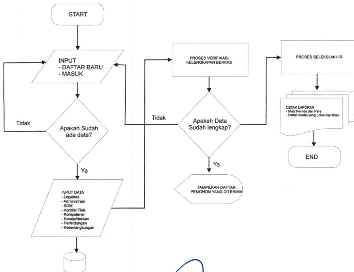
Alur Sistem Aplikasi SIMAPORA
